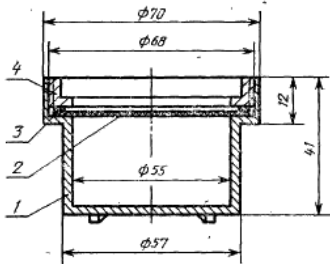
Диффузионная ячейка для гравиметрического метода
