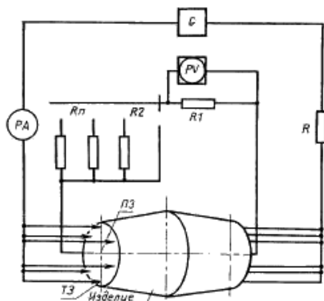
G — источник постоянного тока; PA — прибор для измерения тока, PV — прибор для измерения напряжения, R — ограничивающий резистор; R1—Rn — резисторы делителя напряжения; TZ — токовый зонд; ПЗ — потенциальный зонд
