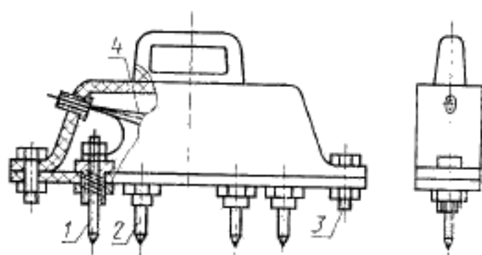
Схема четырехзондового датчика
