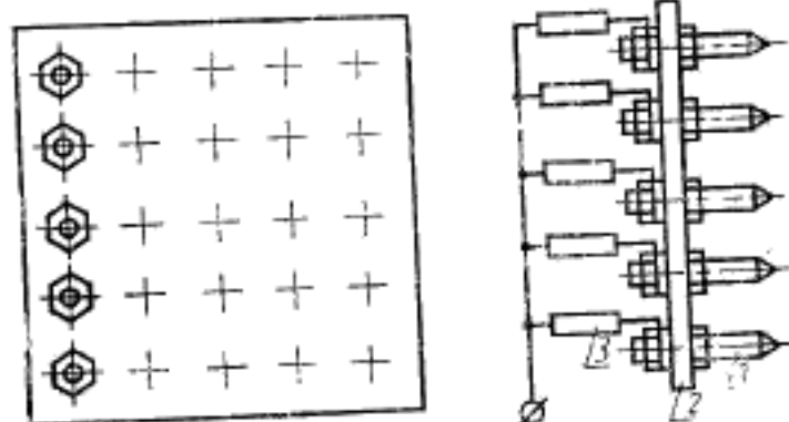
Схема датчиков токовых зондов
