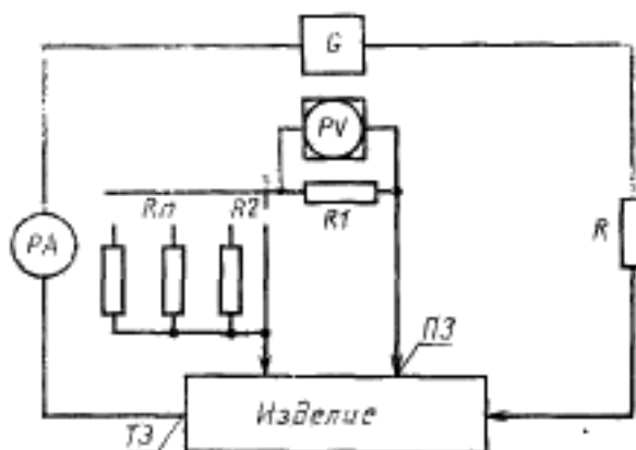
G — источник постоянного тока; PA — прибор для измерения тока; PV — прибор для измерения напряжения; R — ограничивающий резистор; R_1 — R_n — резисторы делителя напряжения; T_3 — токовый зонд; \Pi_3 — потенциальный зонд.
