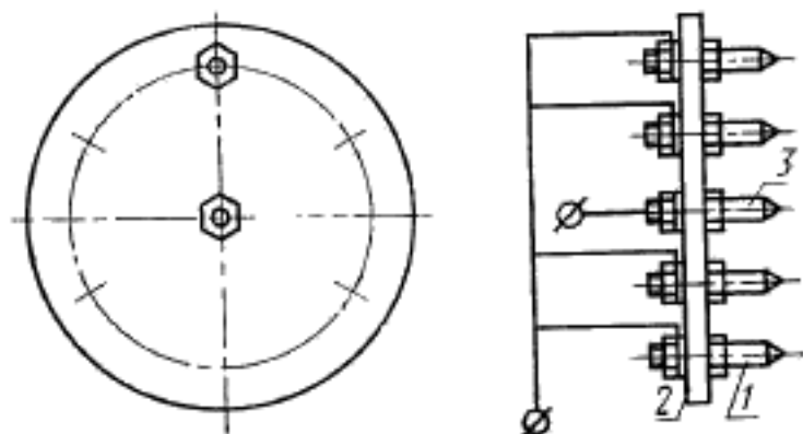
Схема комбинированного датчика
