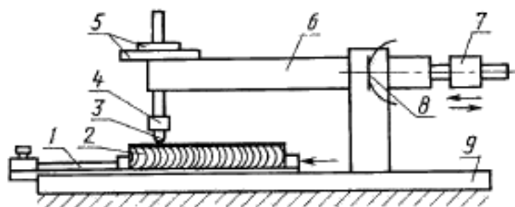
1—жеретка; 2—испытуемый образец; 3—игла; 4—держатель иглы; 5—груз; 6—коромысло; 7—противовес; 8—центр вращения коромысла; 9—подставка
