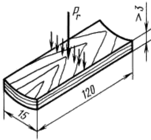
P_r — действие силы удара в радиальном направлении
