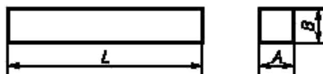
Рисунок А.1 — Размеры образца для испытания на ударный изгиб
