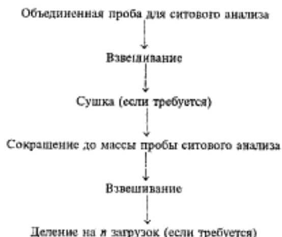
Рисунок 1 — Схема подготовки объединенной пробы к ситовому анализу
