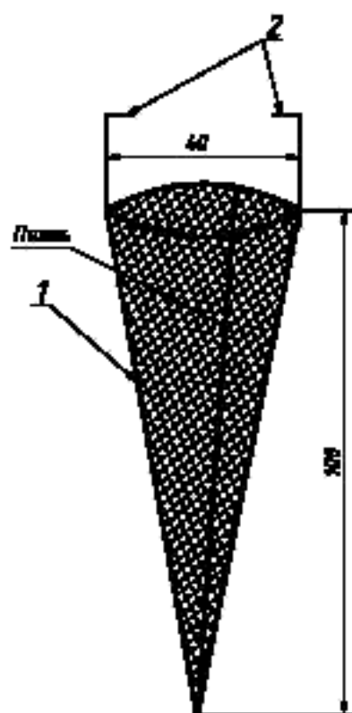
Колпачок для фильтра
