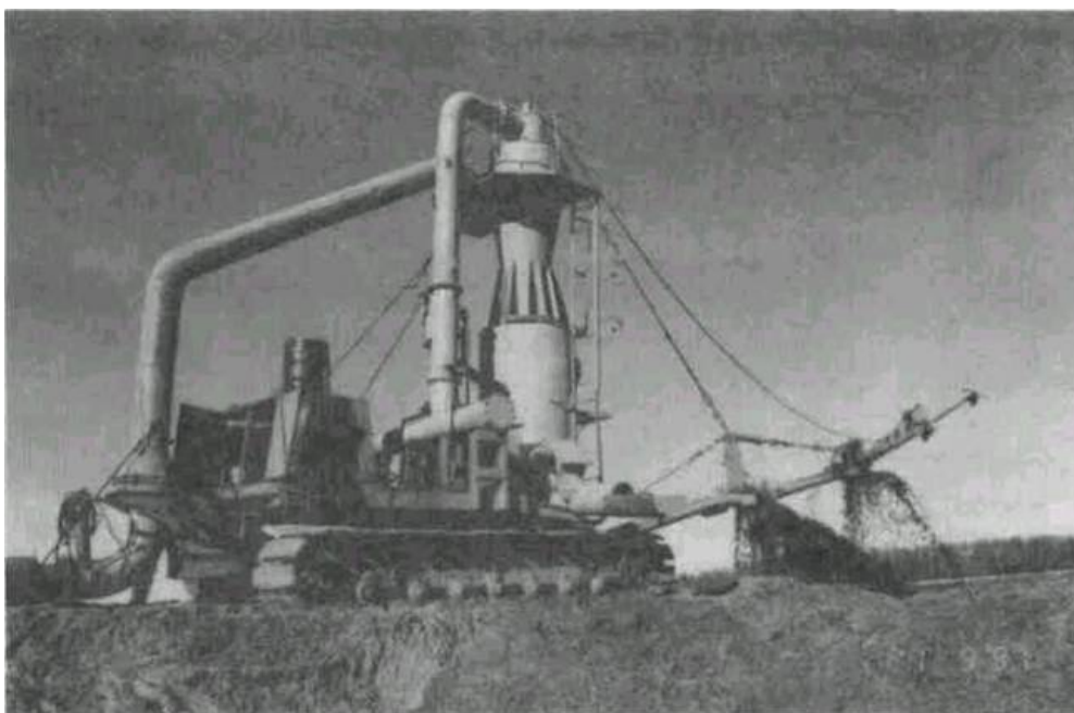
Стелитель-грунтоукладчик СГУ-2000
