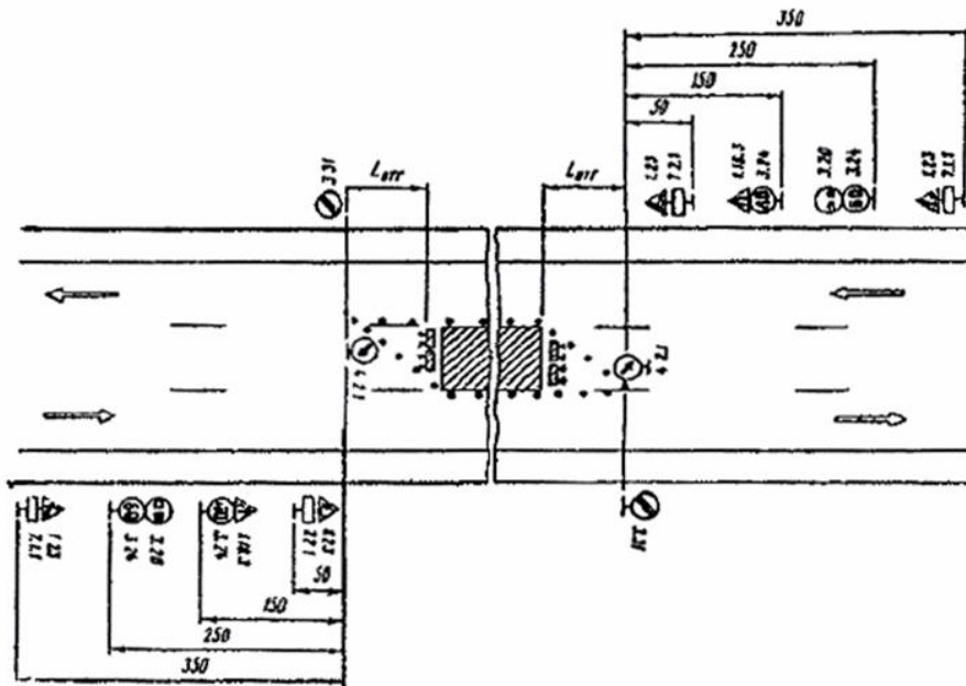
Рис. 3.5. Организация движения и ограждение места дорожных работ, выполняемых на средней полосе движения трехполосных дорог
