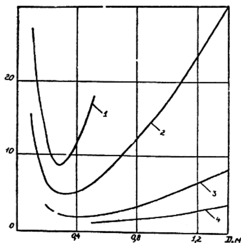
Рис. 2. Зависимость времени прокачки воды с температурой T_{\varepsilon}^* = 50^\circ\text{C} для эталонного трубопровода от его диаметра при суммарной производительности наполнительных агрегатов Q, \text{ м}^3/\text{ч} :
