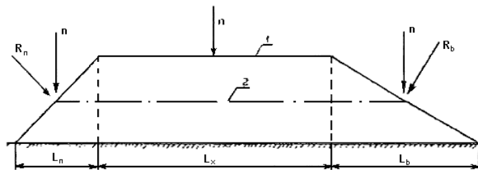
Рисунок 7.2 - Плановое положение искусственного свободного песчаного пляжа:
