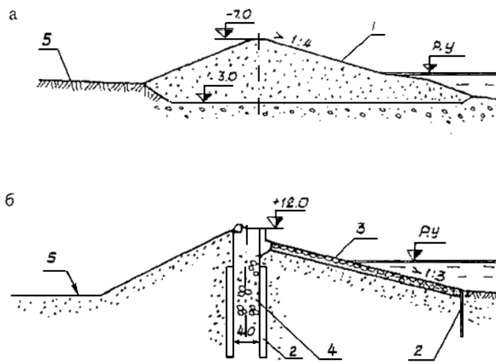
Рисунок 7.7 - Оградительные дамбы с укрепительными откосами:
