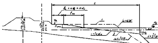
Рисунок 7.6 - Схема волногасящей бумы из несортированной горной массы с геометрически изменяемым профилем:
