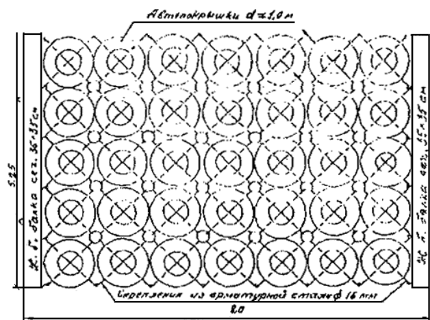
Рисунок 7.28 - Конструкция защитного "ковра" из автопокрышек
