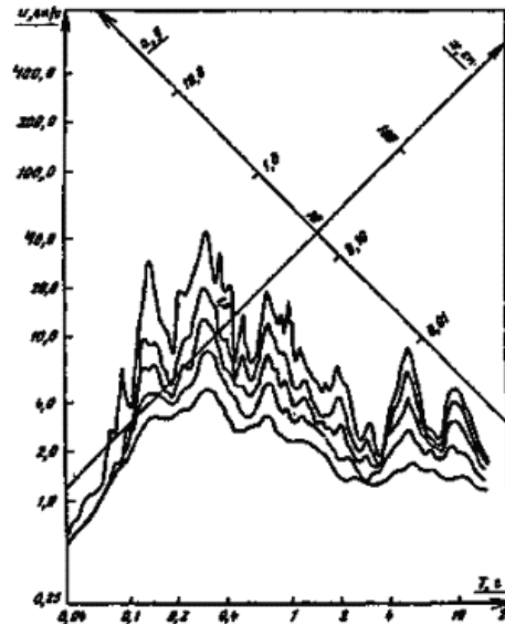
Рис. 1.4. Образец спектра реакции трехкоординатной сетке
