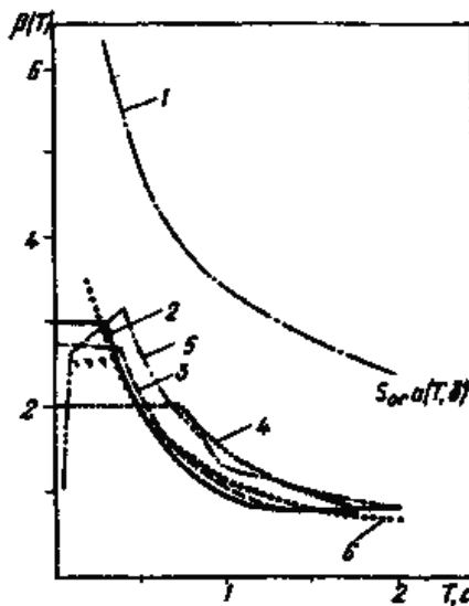
Рис. 5.1. Коэффициенты динамичности линейных осцилляторов при затухании \delta , равном 5%
