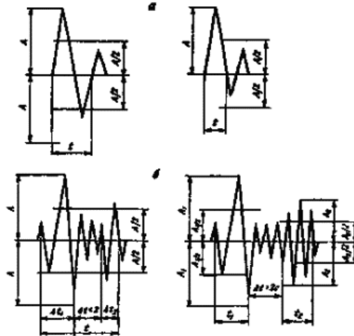
Рис. 1.3. Схема измерения ширины импульса:
