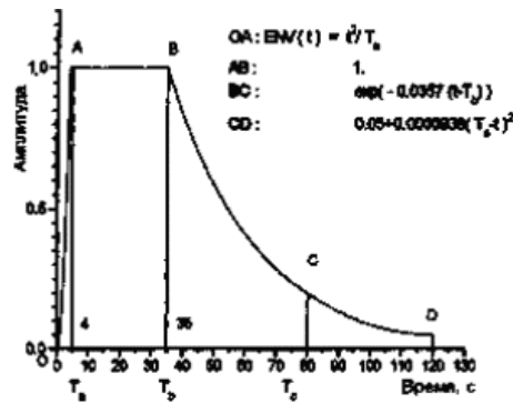
Рис. 3. Форма амплитуды огибающей колебаний
