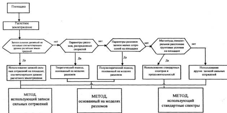
Рис. 1. Схема алгоритма определения исходных сейсмических воздействий
