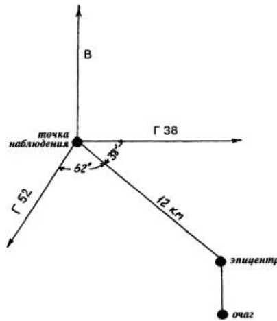
Рис. 1.2. Схема обозначения составляющих, принятая на акселерограммах
