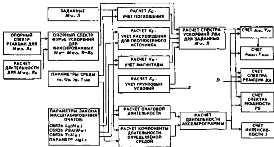
Рис. 2.2. Блок-схема алгоритма моделирования параметров колебаний фунта
