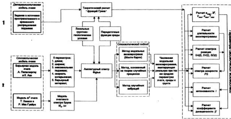
Рис. 2.1. Блок-схема определения параметров сейсмических колебаний груша методами, основанными на модели разлома"
