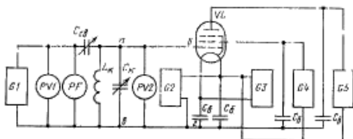
G1 —генератор напряжения; PV1 , PV2 —вольтметры переменного тока; PF —измеритель частоты; C cb —конденсатор связи; L k —катушка индуктивности контура; C k —конденсатор контура; G2 , G3 , G4 , G5 —источники питания; VL —испытываемая лампа; C 6 —блокировочный конденсатор
