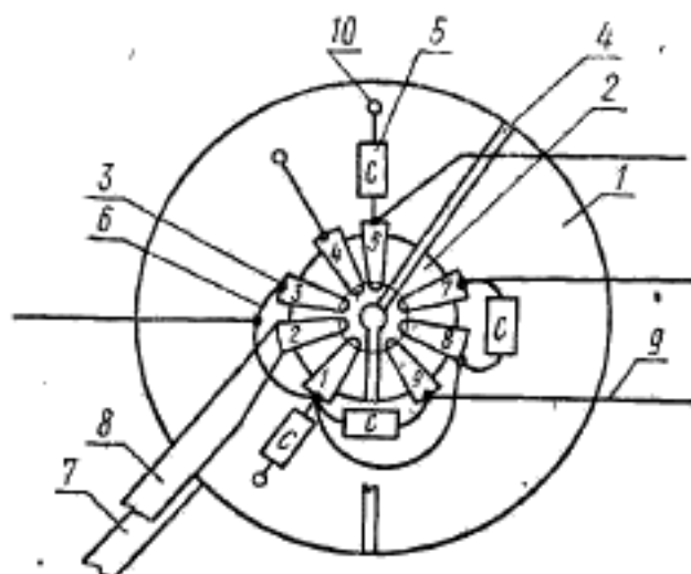
1—проводящая заземляющая плата; 2—ламповая панель; 3—лесточка ламповой панели; 4—экран между электродами; 5—конденсатор; 6—монтажный проводник; 7 и 8— шины; 9—проводник к источнику питания; 10—пайка
