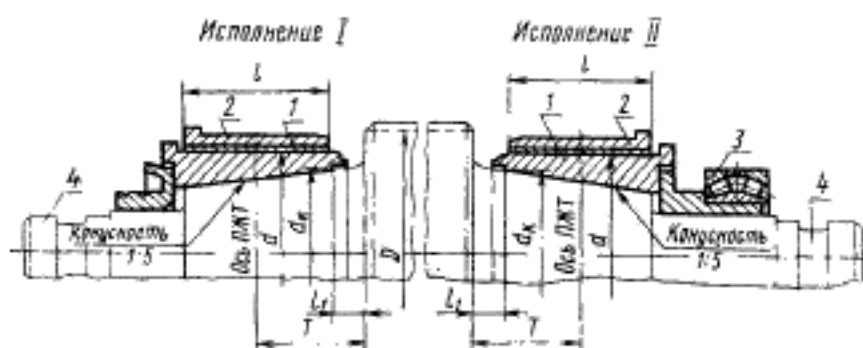
Черт. 4
