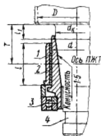
Черт. 6
