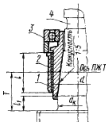
Исполнение II
