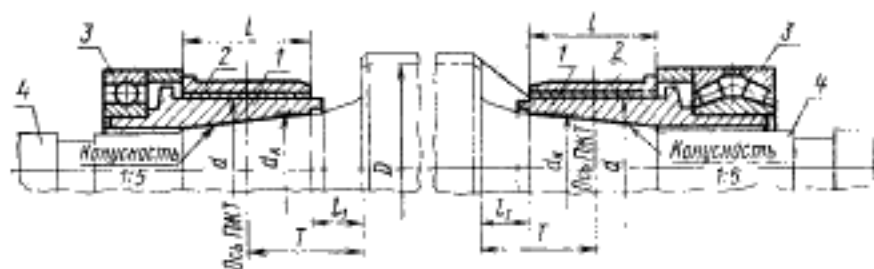
Черт. 3
